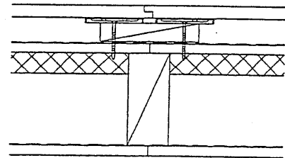
④本実・合いじゃくり目地
