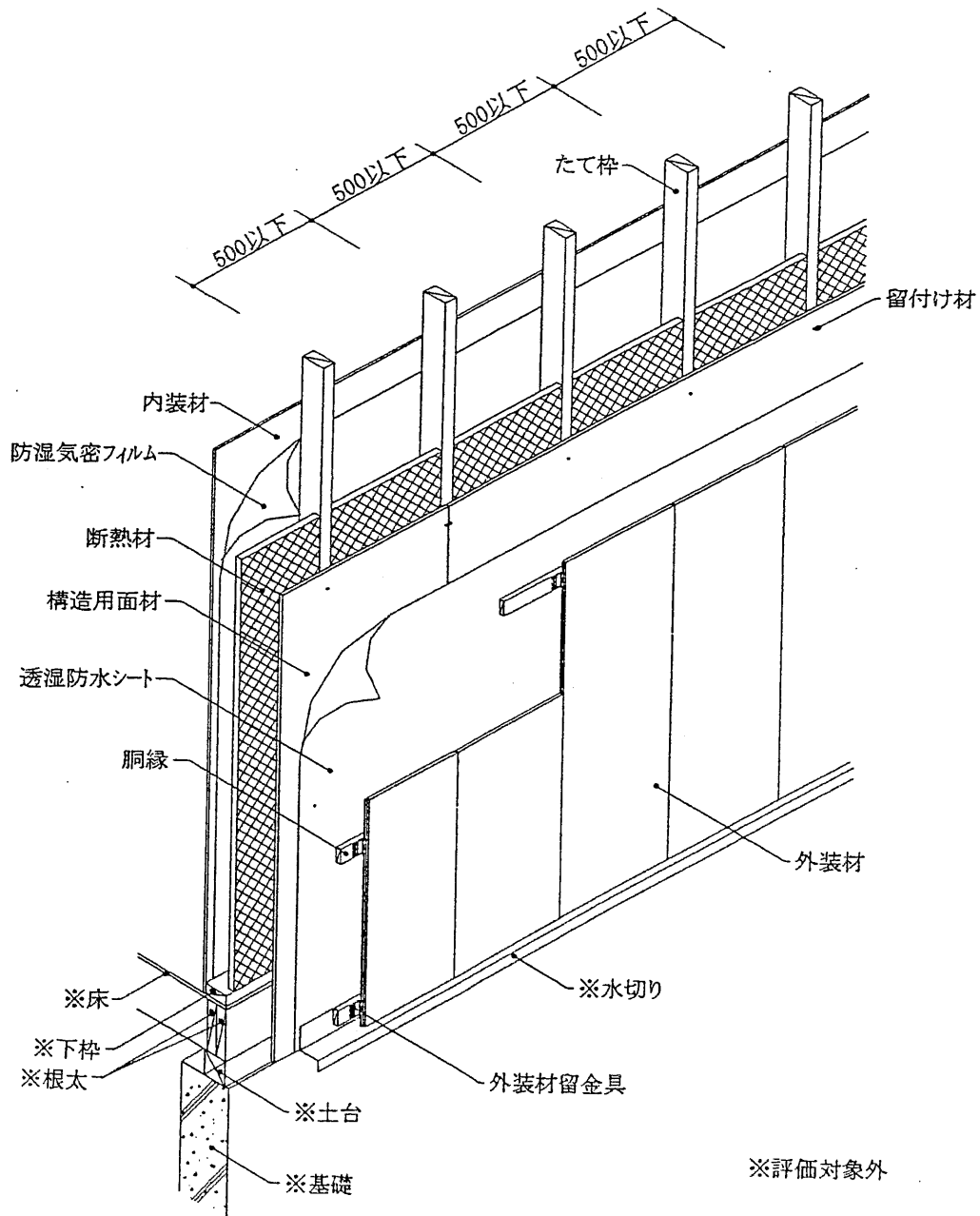
透視図
