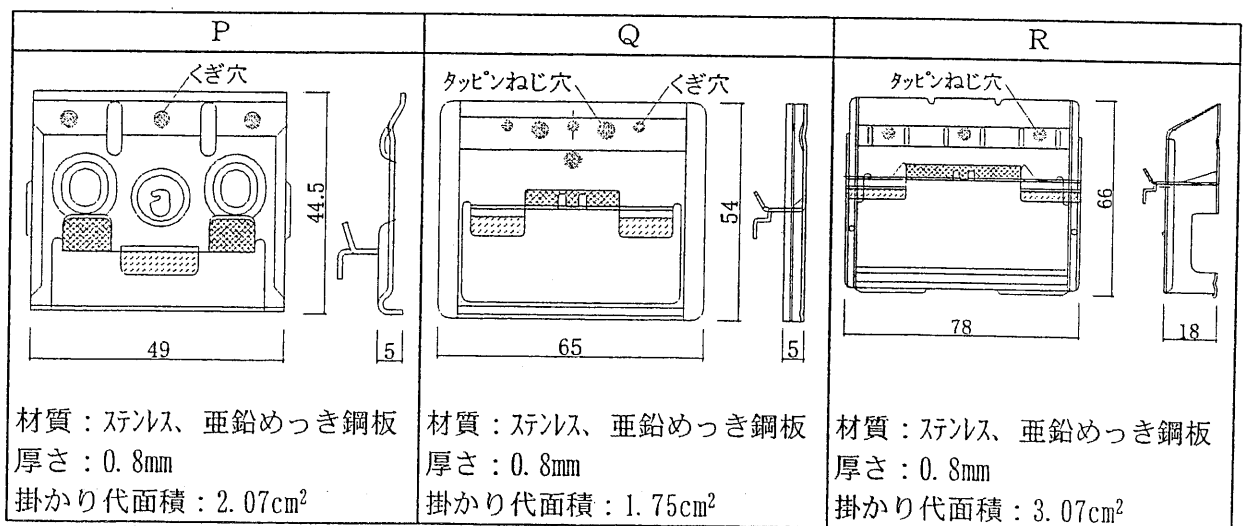
図8 構造説明図
