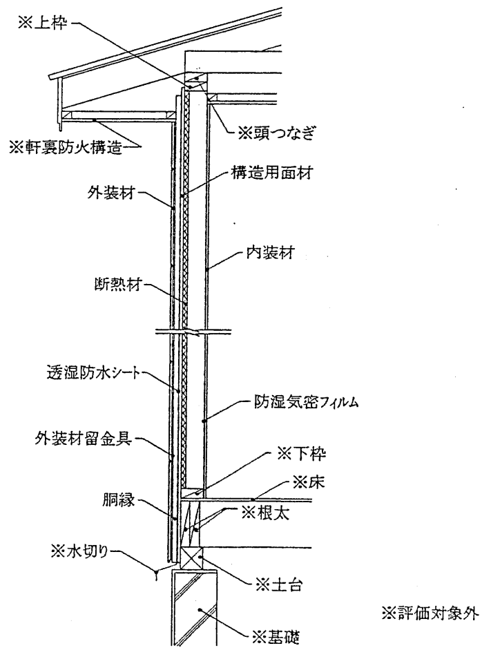
鉛直断面図
