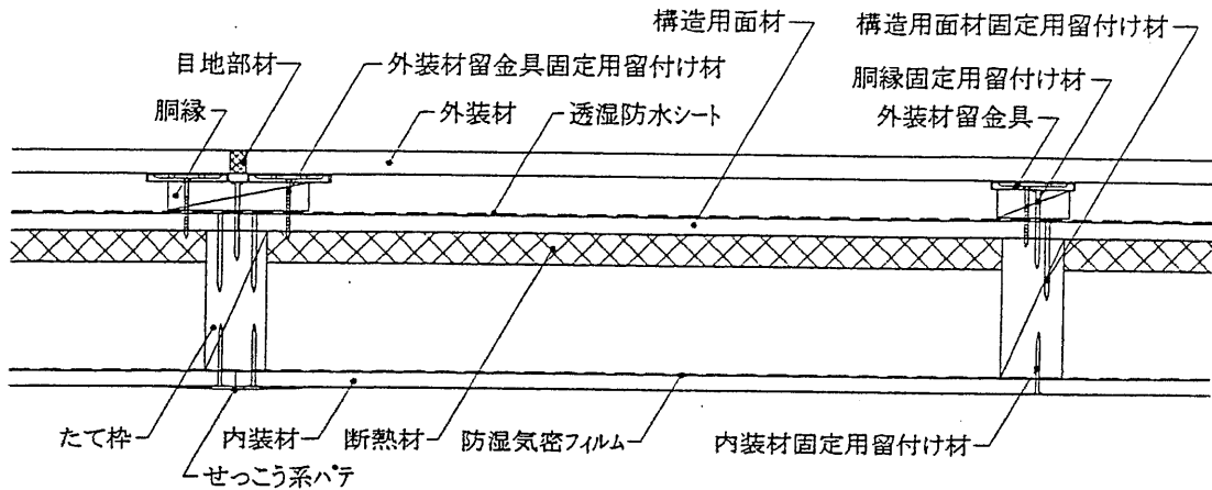
水平断面図
