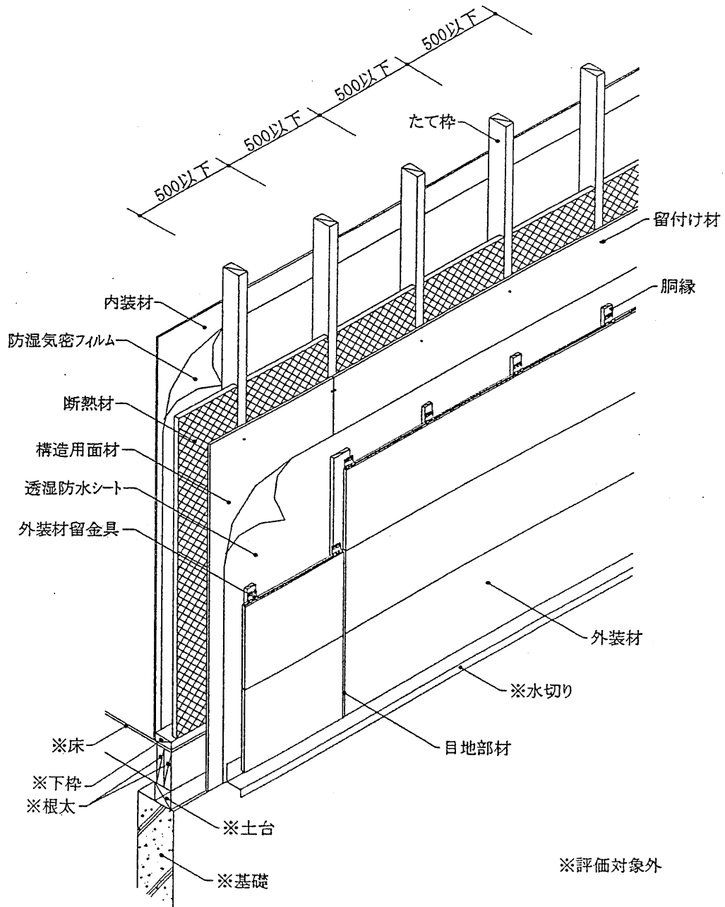
透視図
