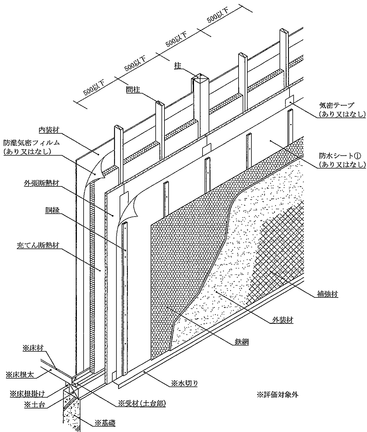
透視図 (欠き込み真壁造) (構造用面材なし・下地材なし・充填断熱材あり仕様)
